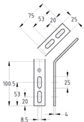
Szerelőszelet 45°
