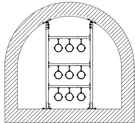
Boltíven vagy kerek kábelcsatornáknál és aknáknál történő konzolszereléshez
