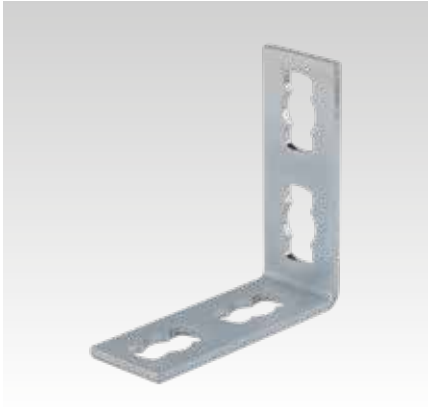
MPR-szerelőszeget 90° 2+2 S+ típus
