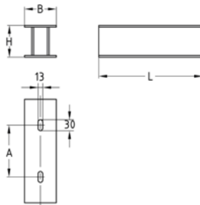
Q80, Q150 profilokhoz Elnagyolt tervrajz (az eredeti kivitel eltérő lehet)
