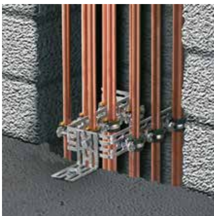
Szerelés aknában: Az M8 Stabofix® csavarral is szerelhetjük a csőbilincseket
