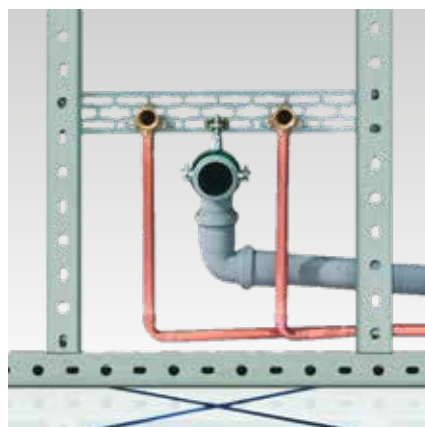
Fal előtti szerelés: Fal előtti szerelés Stabofix® és MPC-rendszer sínek felhasználásával
