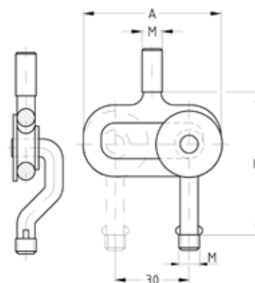
Görgős fül egy MÜPRO csavaros csőbilinccsel
